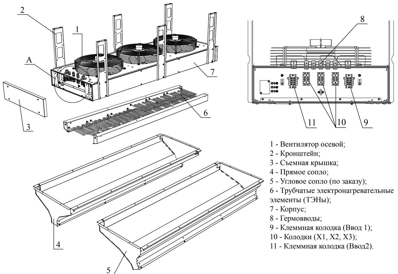
Рисунок 1. Воздушно-тепловая завеса
